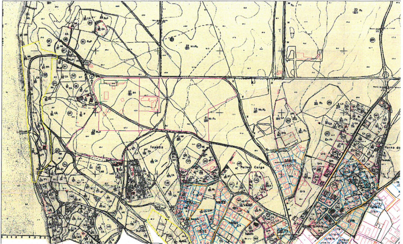
Planta 2: Planta cadastral da área.
